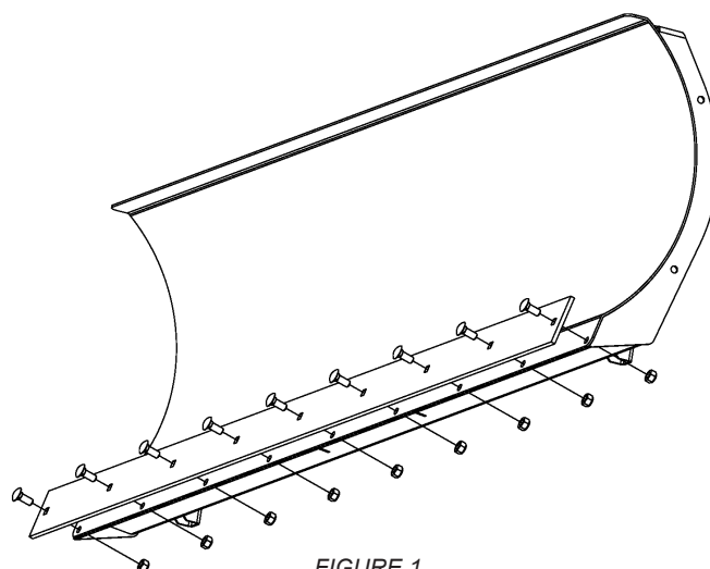
FIGURE 1 INSTALLATION DE LA BARRE D'USURE
